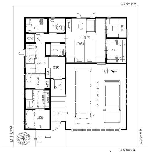
配置図兼 1階平面図
