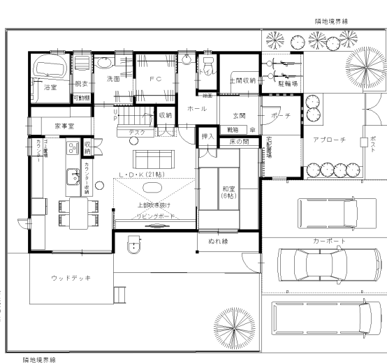
配置図兼 1階平面図
