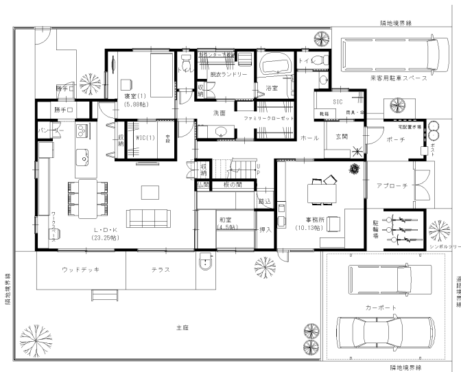
配置図兼 1階平面図
